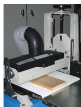
Calibrage "Fermé" 1 seul passage, largeur de bois inférieur à 410 mm.
